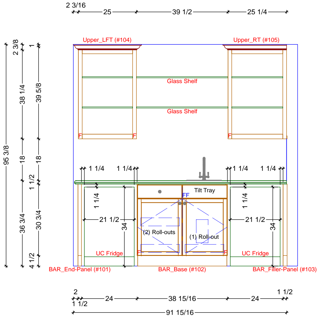
1 BAR ELEVATION - NORTH SCALE: 1/2" = 1' 0"
