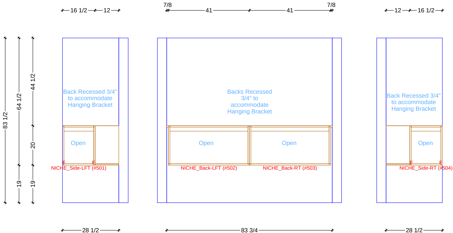
1 NICHE ELEVATION - LEFT SCALE: 1/2" = 1' 0"
