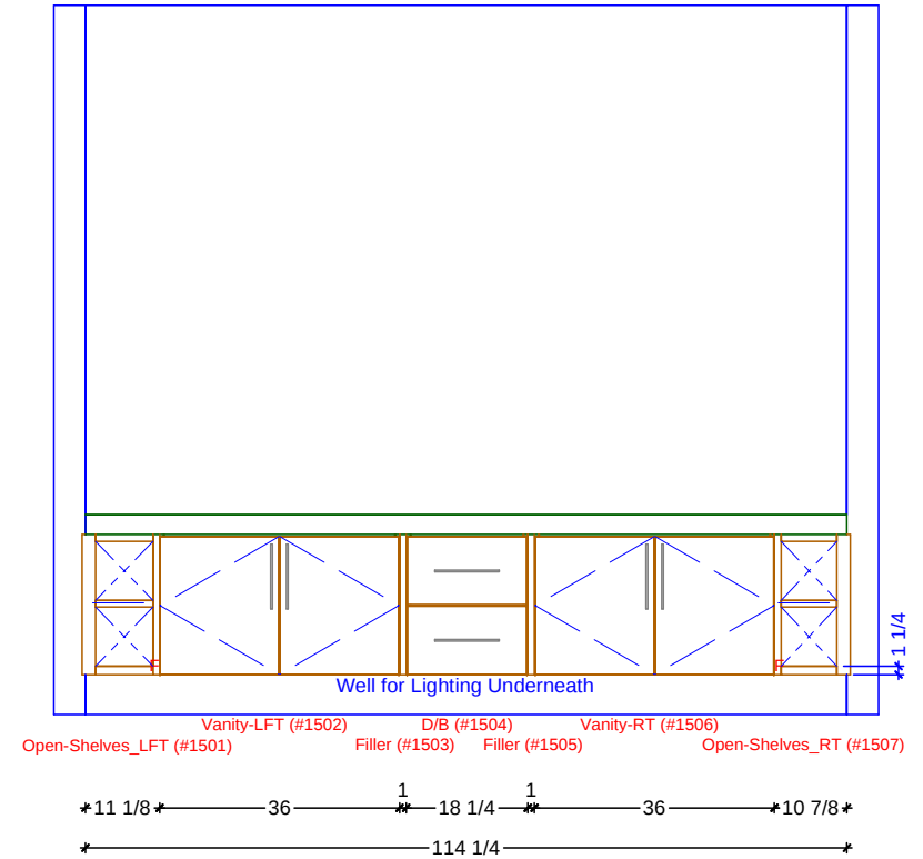
1 ELEVATION VIEW SCALE: 3/8" = 1' 0"
