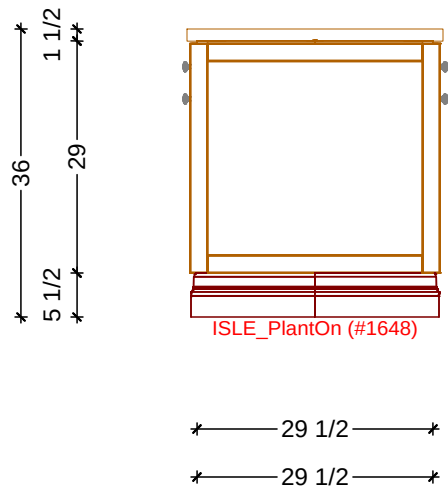
I ELEVATION SCALE: 3/8" = 1' 0"
