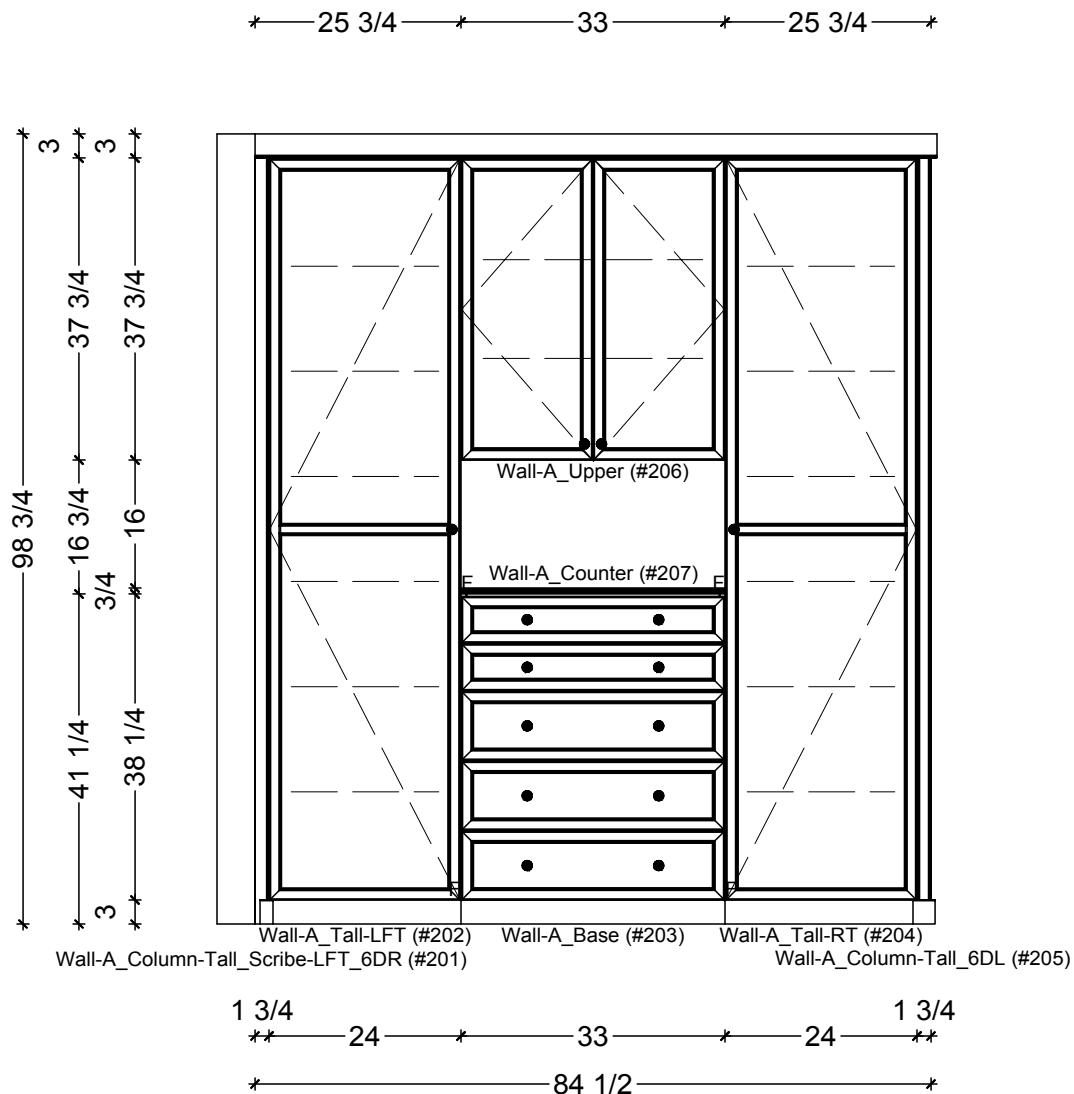
1 WALL-A ELEVATION SCALE: 1/2" = 1' 0"
