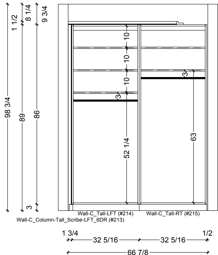
2 WALL-C ELEVATION SCALE: 1/2" = 1' 0"
