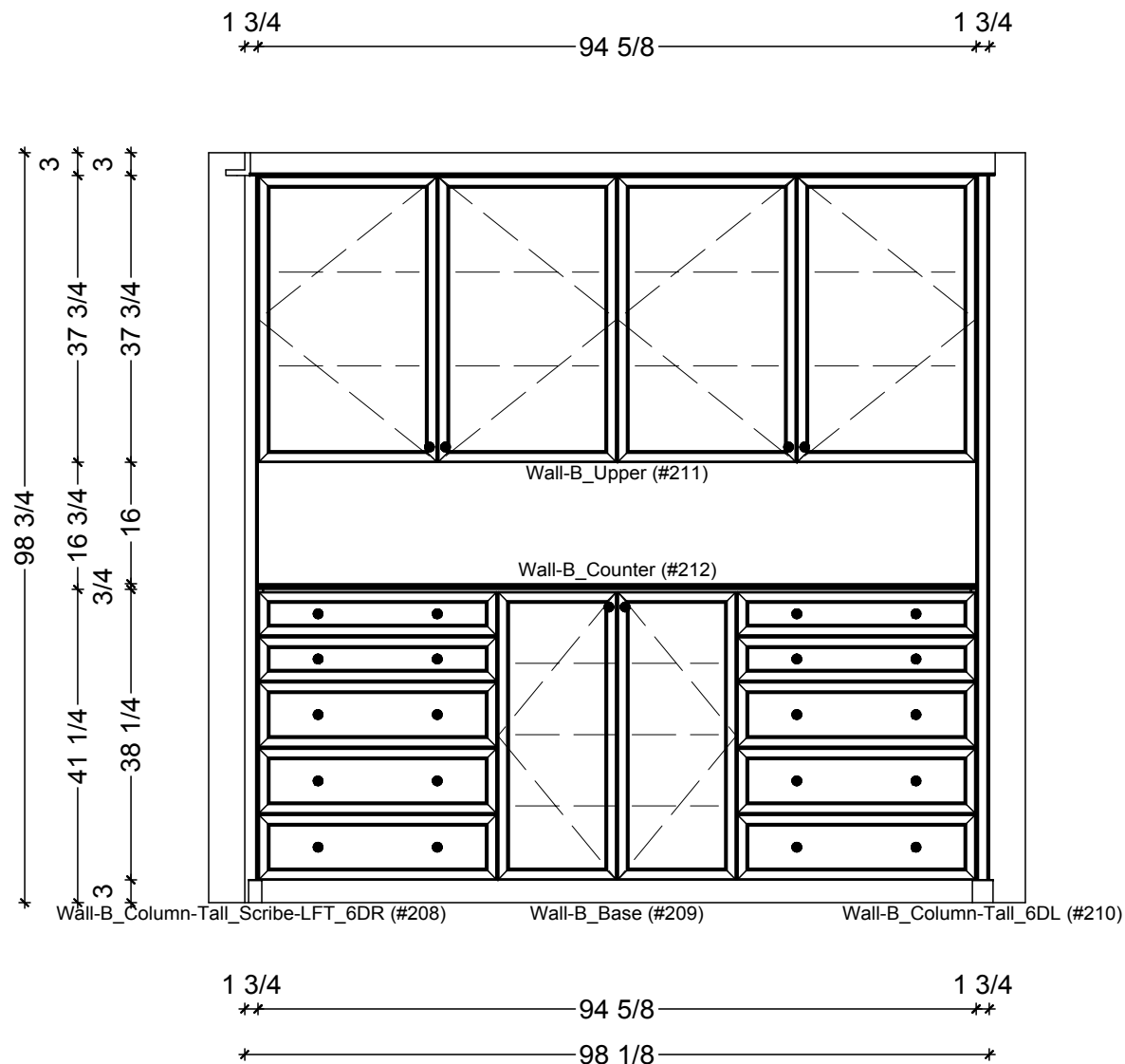
1 WALL-B ELEVATION SCALE: 1/2" = 1' 0"
